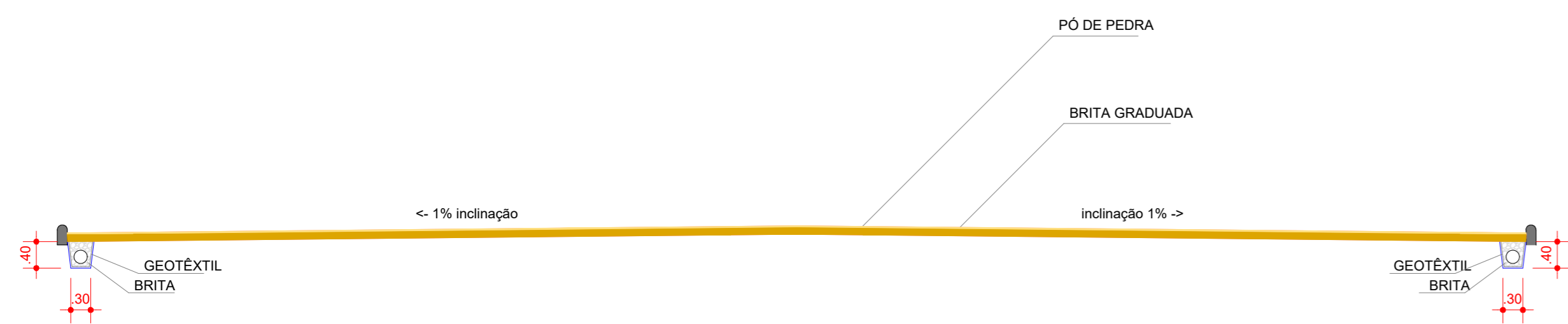
DETALHE 1 CORTE TRANSVERSAL ESQUEMÁTICO - DRENAGEM ESCALA 1:125
