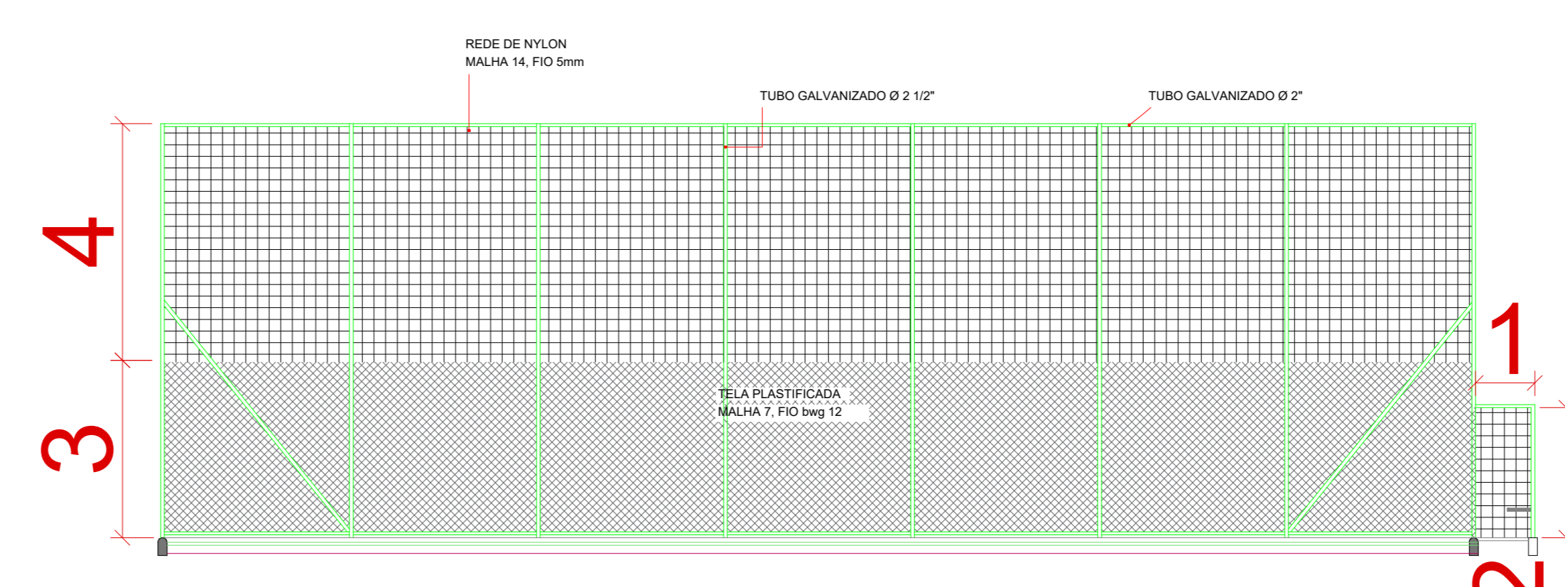
CORTE TRANSVERSAL ESCALA 1:125
