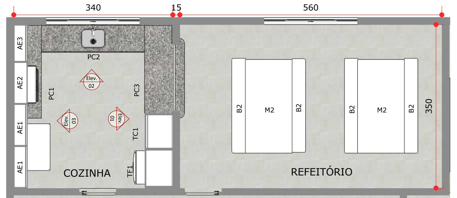
LAYOUT COZINHA E REFEITÓRIO esc.: 1/50
