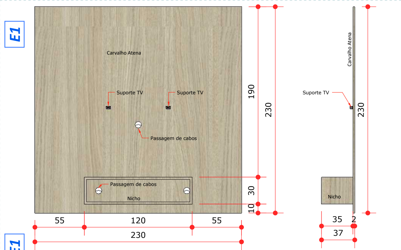
VISTA FRONTAL E1 esc.: 1/25
