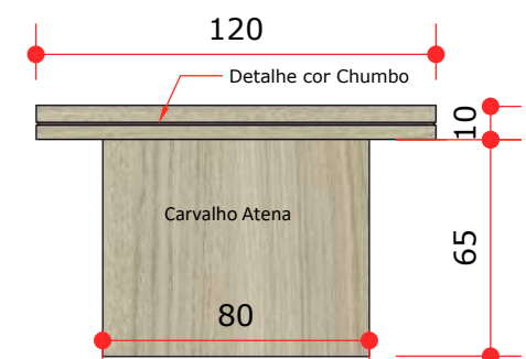
VISTA LATERAL M1 esc.: 1/25
