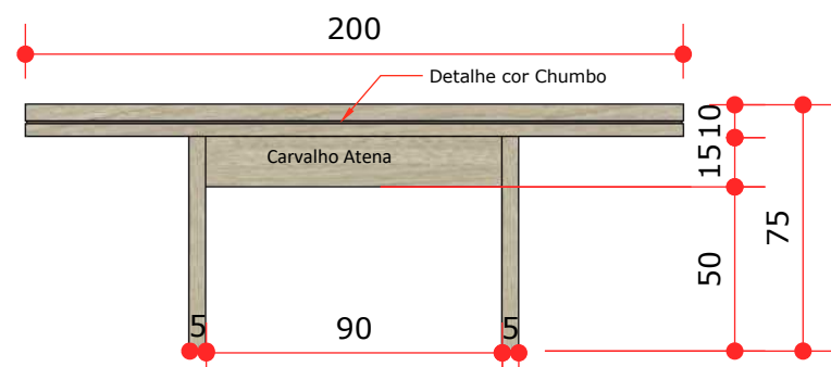
VISTA FRONTAL M1 esc.: 1/25
