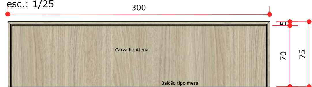
VISTA FRONTAL M5 esc.: 1/25
