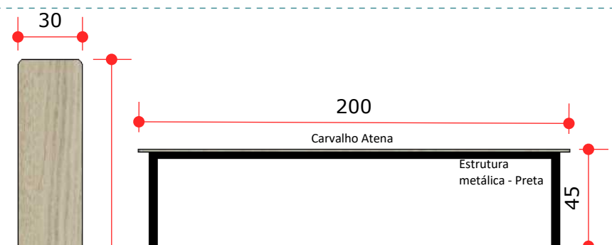
VISTA FRONTAL B1 esc.: 1/25
