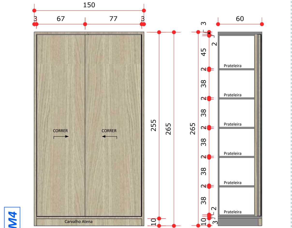
VISTA FRONTAL AM4 esc.: 1/25
