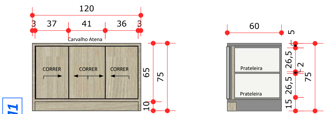
VISTA FRONTAL AM1 esc.: 1/25
