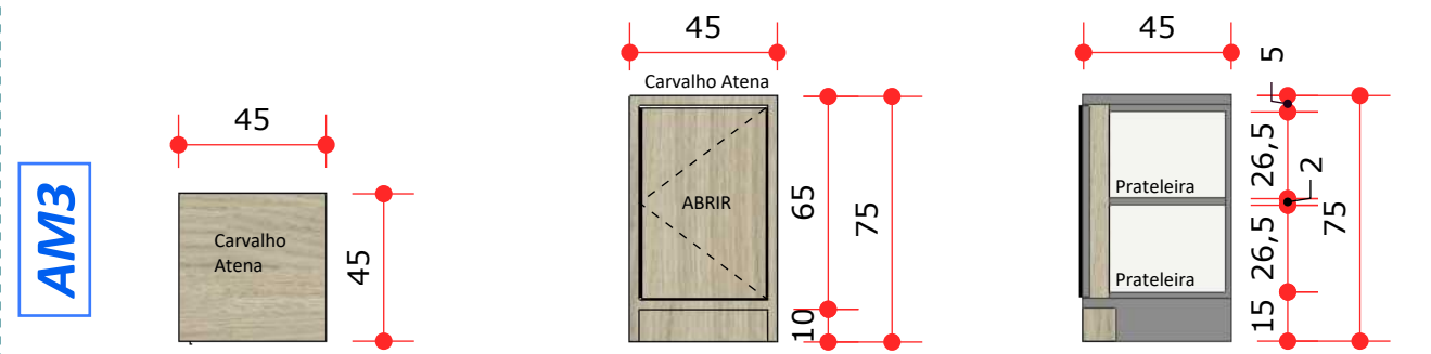
PLANTA BAIXA AM3 esc.: 1/25
