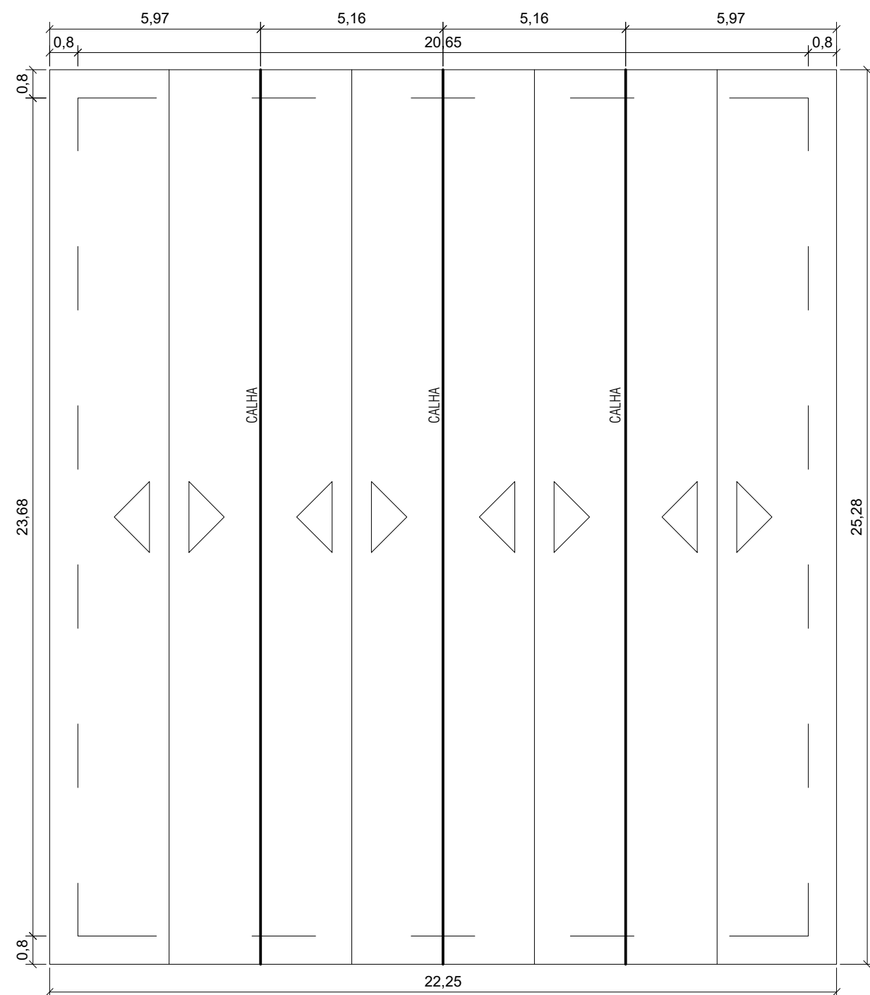
PLANTA DE COBERTURA Esc. 1:150
