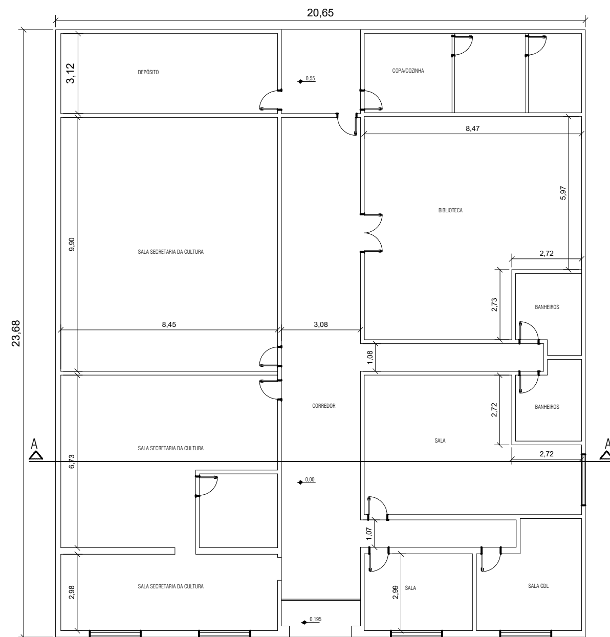
PLANTA BAIXA Esc. 1:150
