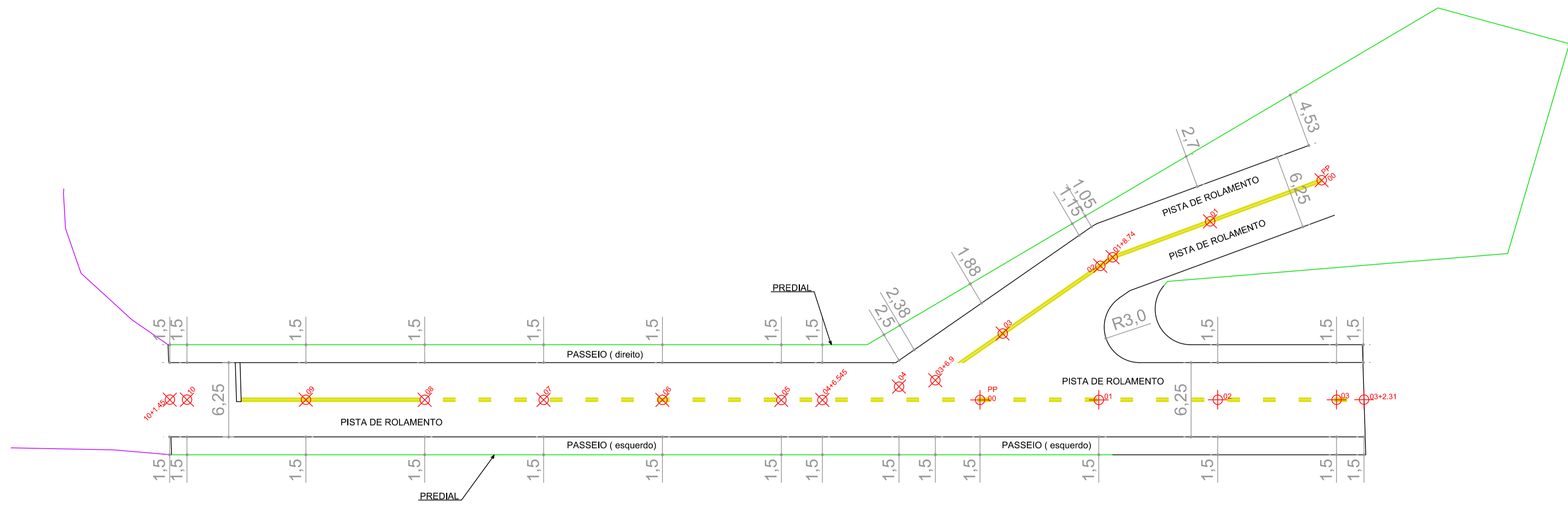
GEOMETRIA PAVIMENTAÇÃO ESCALA 1:250
