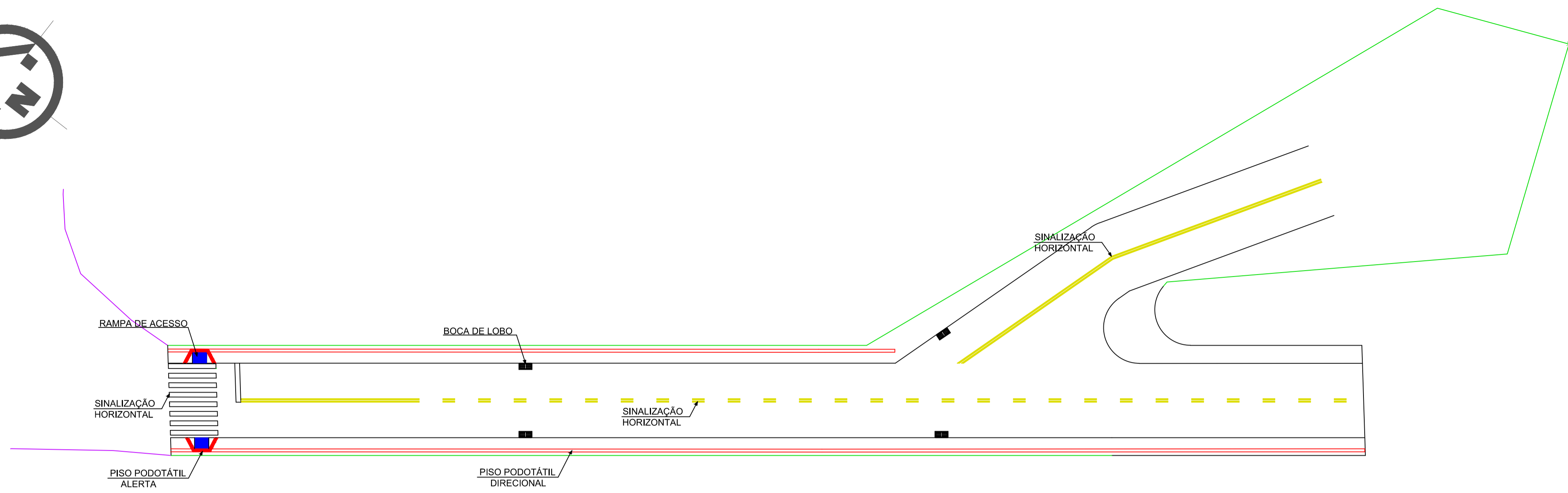
IMPLANTAÇÃO SINALIZAÇÃO HORIZONTAL E VERTICAL ESCALA 1:250
