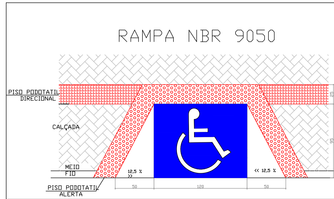
DETALHE RAMPA ESCALA 1:20
