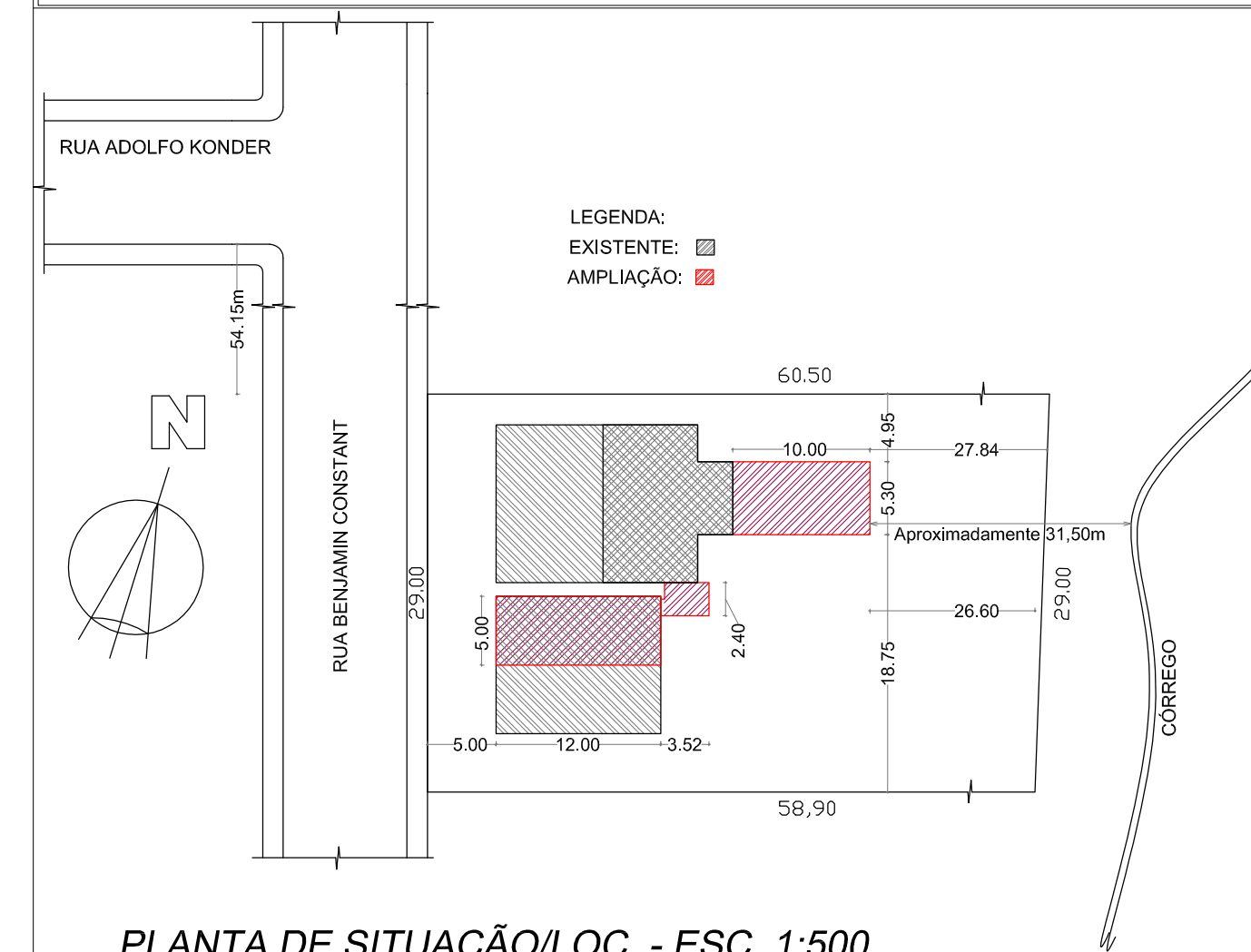
PLANTA DE SITUAÇÃO/LOC. - ESC. 1:500
