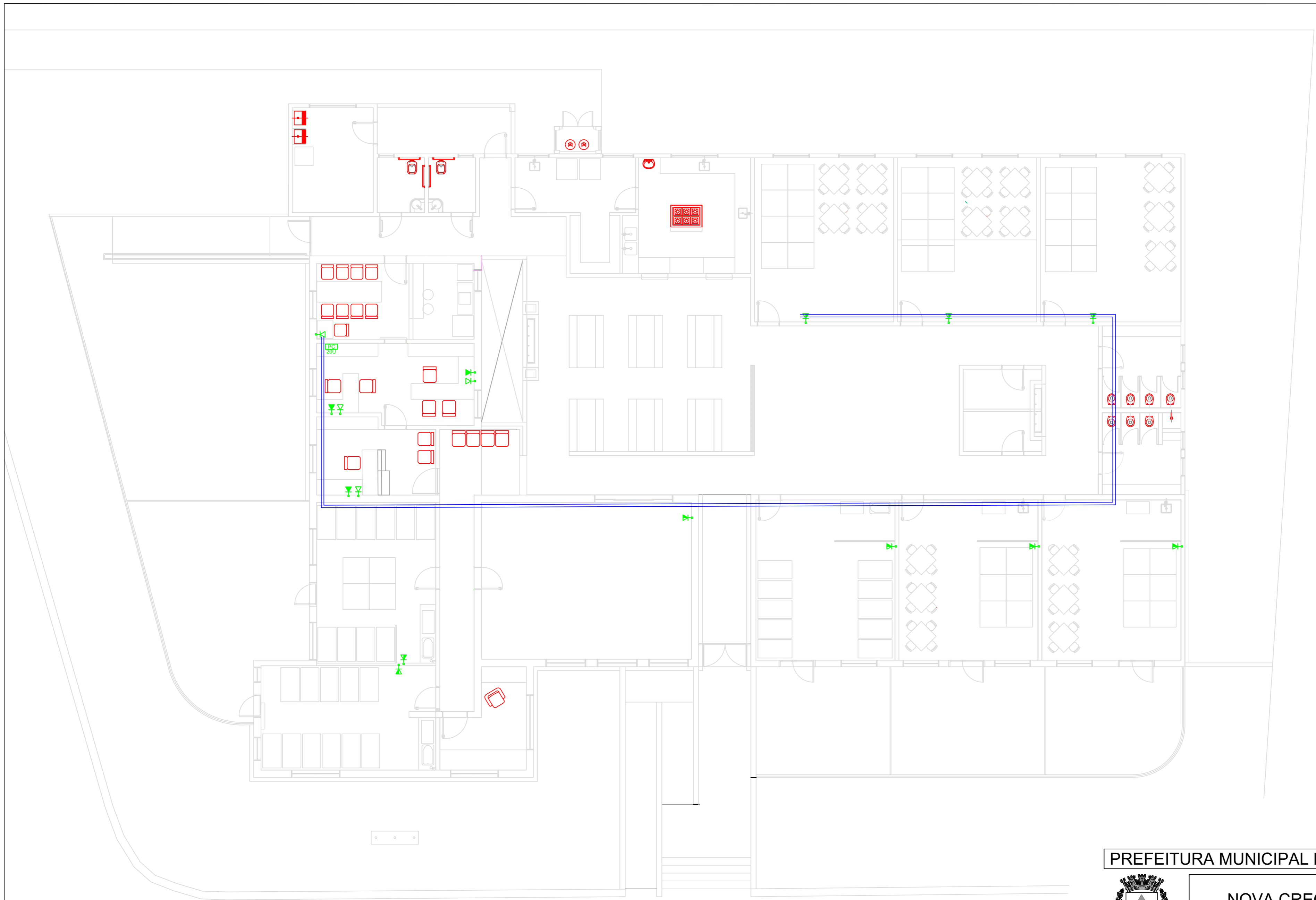
PLANTA DE DISTRIBUIÇÃO TELEFONIA E LÓGICA ESC. 1/100
