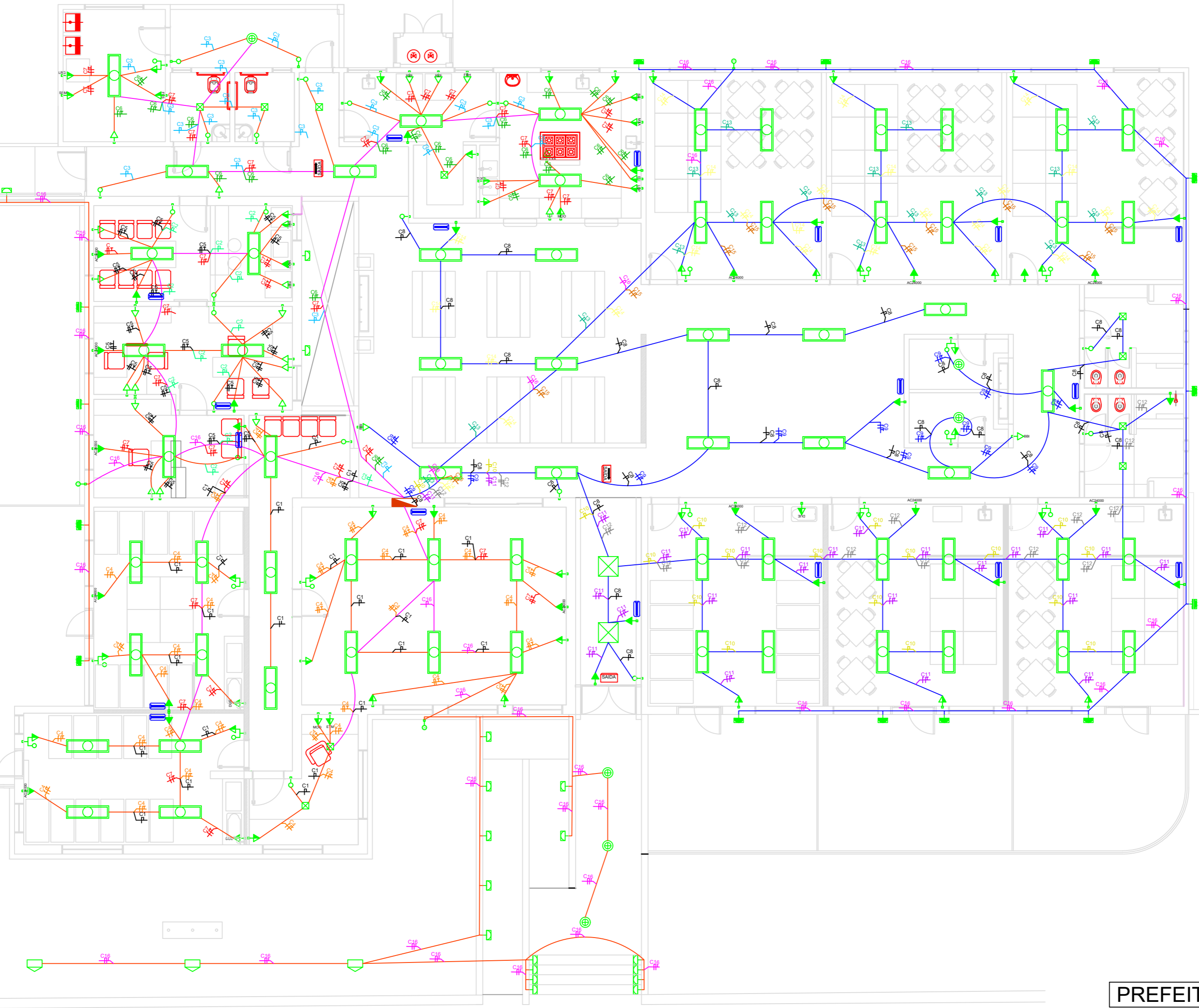
PLANTA DE DISTRIBUIÇÃO ELÉTRICA 500 1/100
