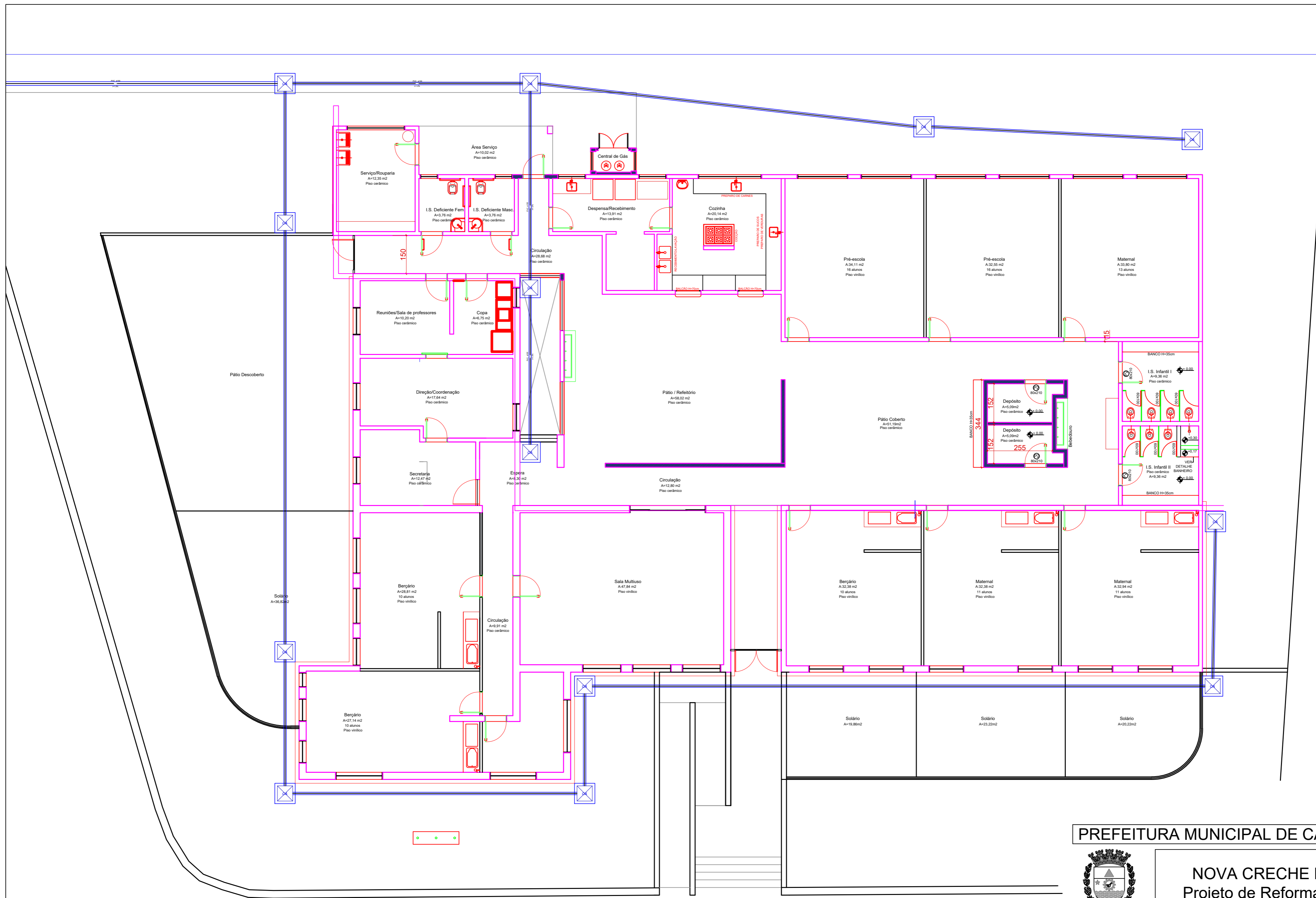
PLANTA DE DRENAGEM PLUVIAL ESC. 1/100
