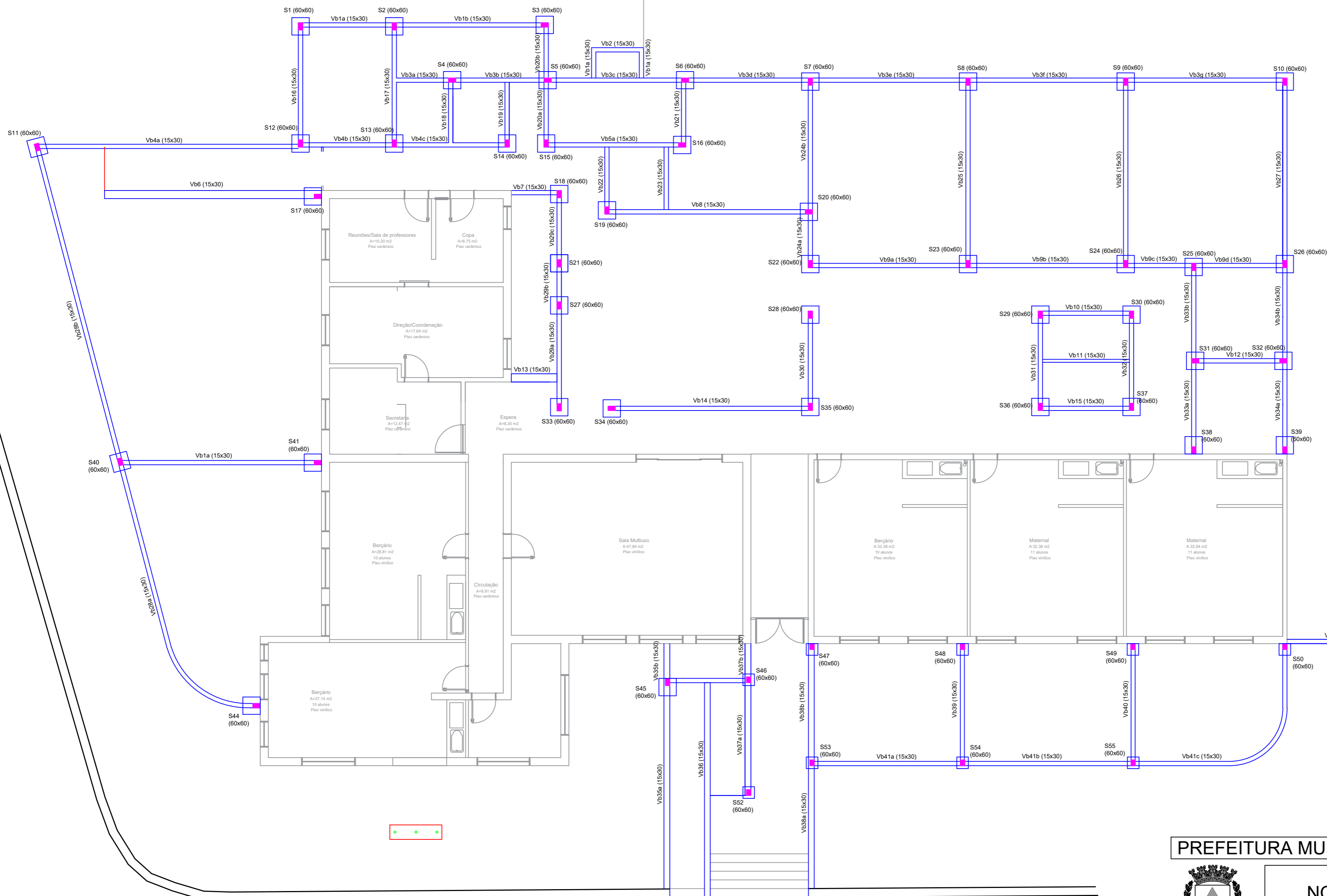
PLANTA DE DISTRIBUIÇÃO DA FUNDAÇÃO
