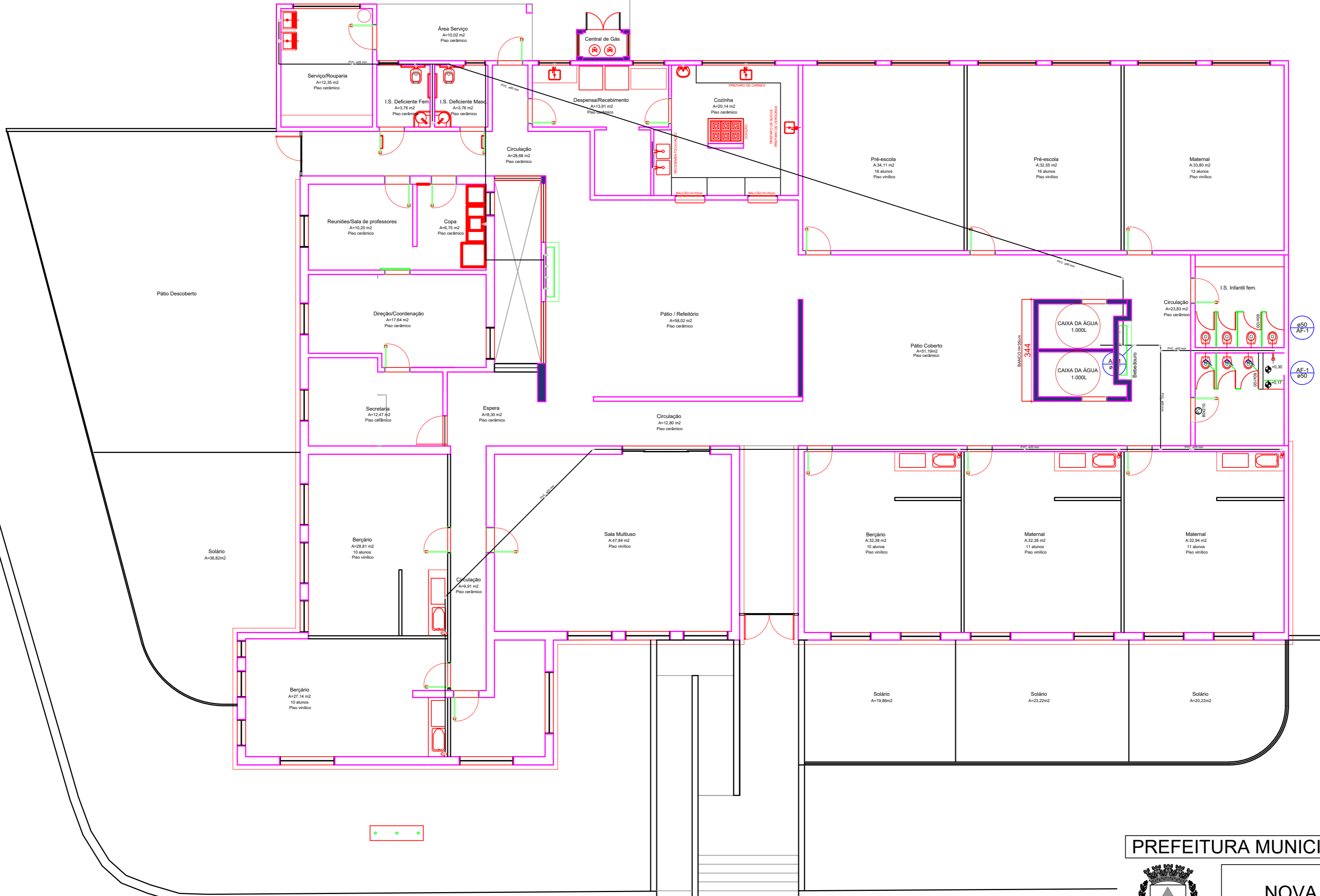
PLANTA DE DISTRIBUIÇÃO DE ÁGUA FRIA ESC. 1/100
